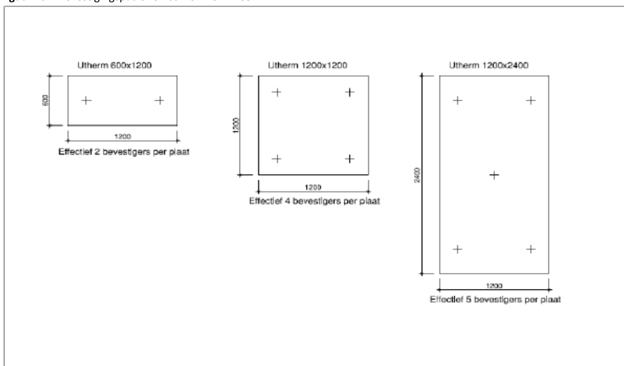
Figuur 2a – Bevestigingspatronen conform SBR 239
